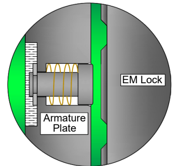
EM Lock De-Energized
