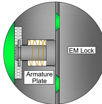
EM Lock Energized
